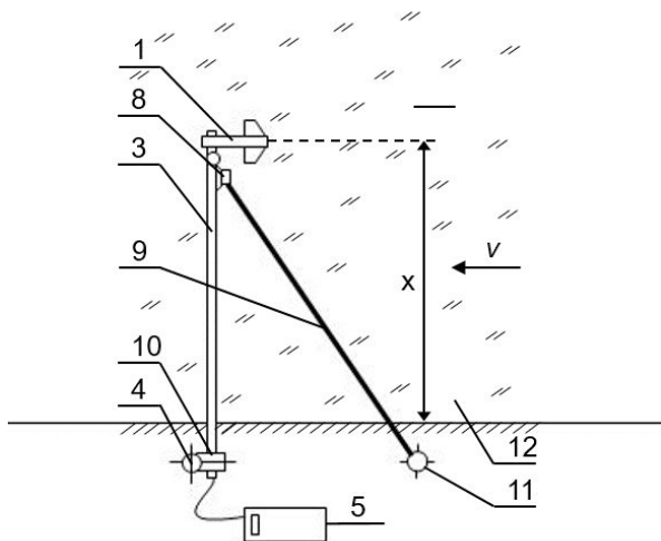
Рисунок 2. Схема измерения скорости потока воды на его поверхности, в зависимости от удалённости от берега X , где 1,3,4,5 — как на Рис.1; 8 — узел крепления троса 9, удерживающего штангу 3 от смещения под действием потока воды; 9 — трос; 10 — рычажное крепление дистанцирующей штанги 3, позволяющее устанавливать датчик скорости 1 вблизи поверхности потока; 11 — опорный столб для крепления троса 3; 12 — поверхность потока воды.
