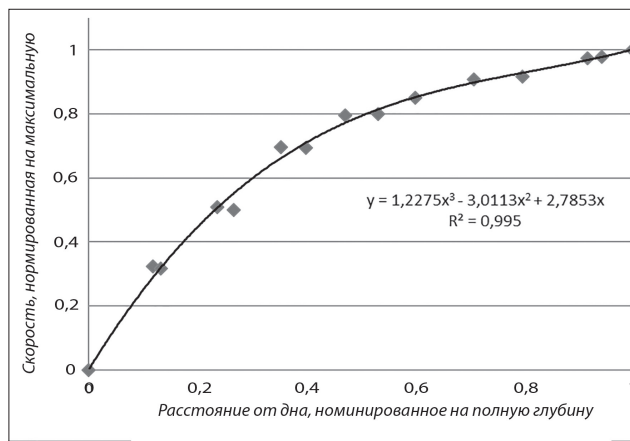
Рисунок 3. Экспериментальные значения скорости воды в речном потоке, от дна к поверхности реки. Глубина и скорость даны в относительных единицах. Приведена аппроксимирующая кривая Y_1(X) .
