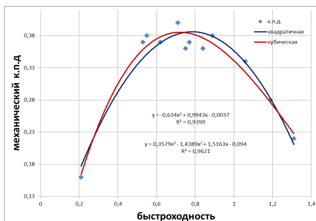
Рисунок 11. Механический к.п.д. турбины
