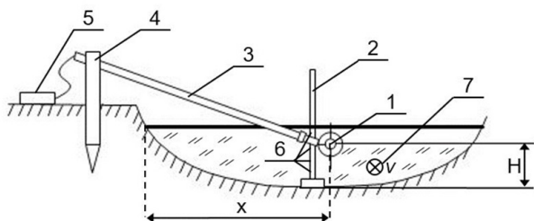
Рисунок 1. Схема измерения скорости потока воды в зависимости от удалённости точки измерения от дна H и от берега X , где 1 — вертушка [2] — типовый измеритель скорости потока по частоте вращения лопастей; 2 — измеритель глубины — столб с опорами 6 для упора штанги 3; 3 — несущая вертушку 1, дистанцирующая штанга, закреплённая на опоре 4; 4 — опорный береговой столб; 5 — измеритель оборотов вала вертушки 1 — датчика скорости потока V ; 6 — опоры для штанги 3 на измерителе глубины 2; 7 — поток воды со скоростью V .
