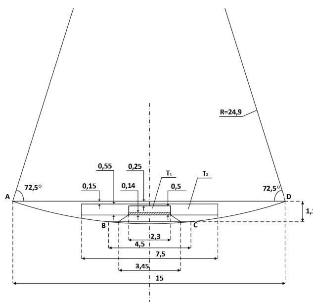
Рисунок 8. Схема положения установки в потоке воды
