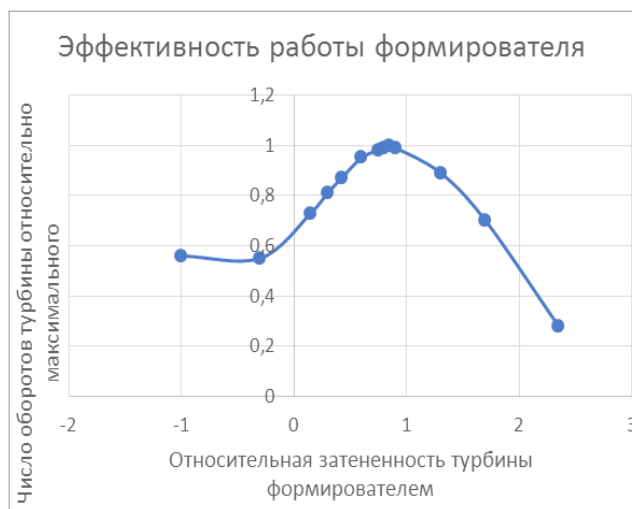
Рисунок 12. Эффективность работы формирователя потока
