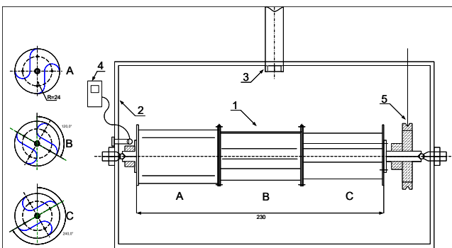
Рисунок 9. Схема размещения поперёк потока модели трёхсекционной турбины 1 диаметром 2R = 48 мм и общей длиной L = 230 мм в закреплённой в корпусе 2 и подвешенной на рычаге 3. Секции турбины A, B, C повернуты на угол 120^\circ относительно друг – друга. Показан электрический вывод 4 с торца турбины на схему, измеряющую угловую скорость турбины и тормозящая вращение нитка 5
