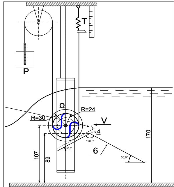
Рисунок 10. Схема измерения мощности турбины
