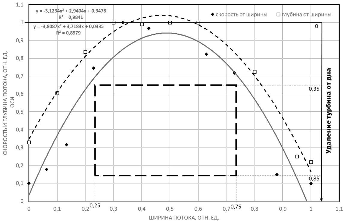
Рисунок 4. Скорость потока V на его поверхности и глубина потока H в зависимости от точки удалённости от берега X , данные в относительных единицах. Показаны аппроксимирующие кривые:
